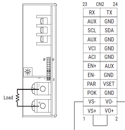
Local Sense (Default Setting)
